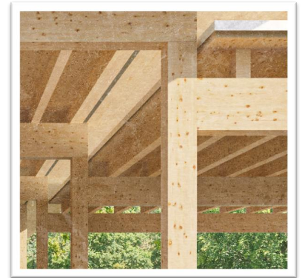
Träger Konstruktion in Fichte
